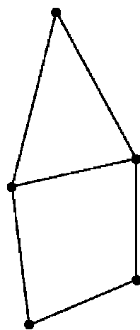
Cepheus
