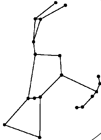
Orion
